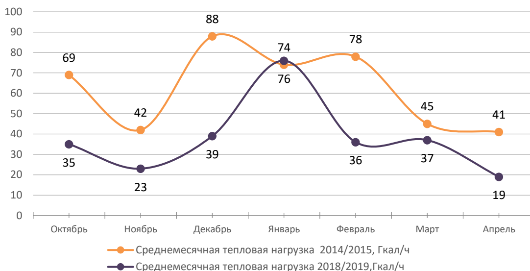
Рисунок 15. График отпуска тепловой энергии по магистральному тепловоду ТВ 16 «Майский»
