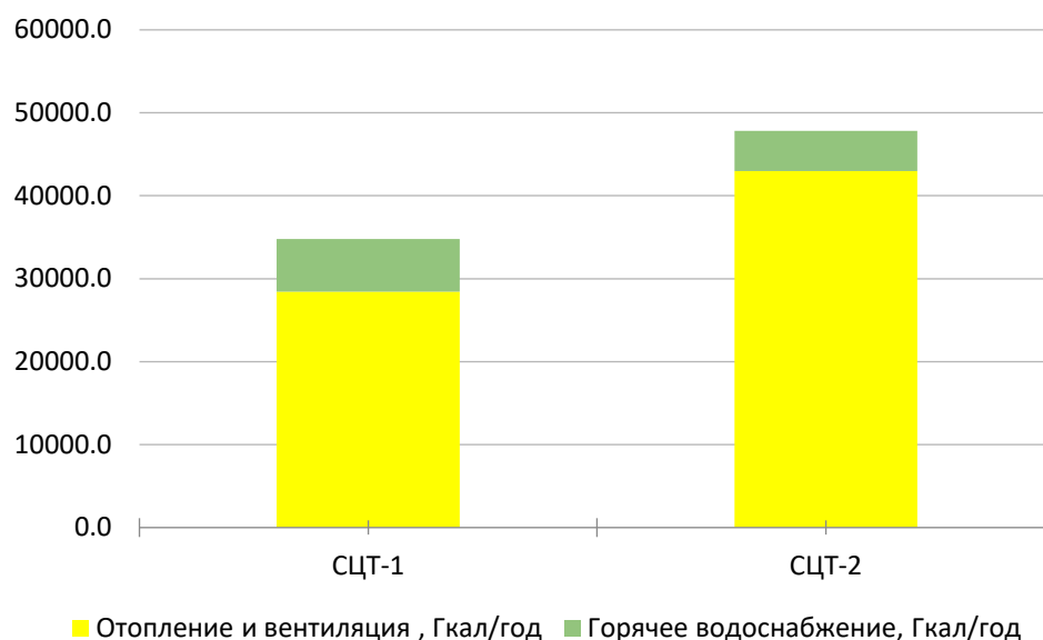
Рисунок 28. Распределение расчетной тепловой энергии по виду нагрузки в расчетных элементах территориального деления Осинковского СП за 2018 г с учетом фактических температур наружного воздуха
