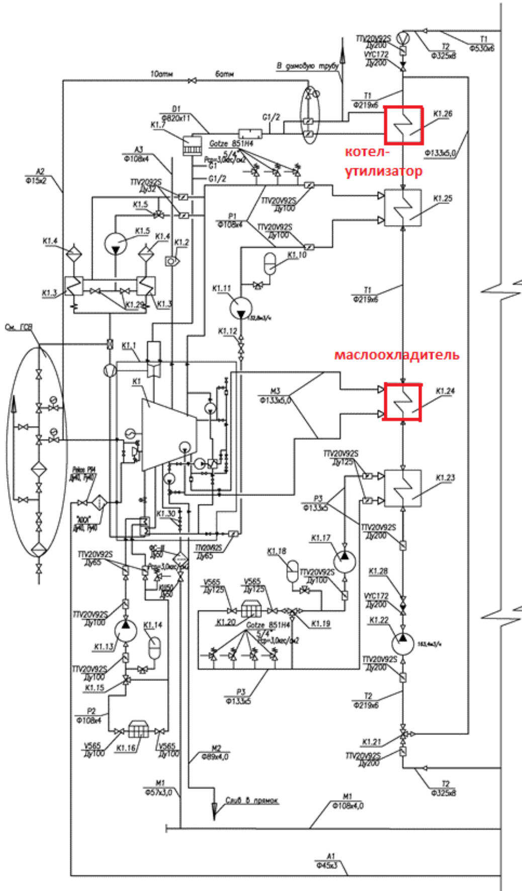
Рисунок 6. Принципиальная схема энергоблока ГПУ ЭЦ «Майский»
